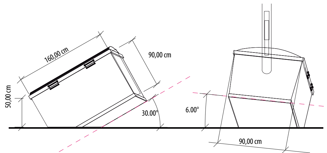
CENTRĀLAIS OBJEKTS. LĀDE. MONTĀŽAS SHĒMA. GABARĪTU MĒRI.
