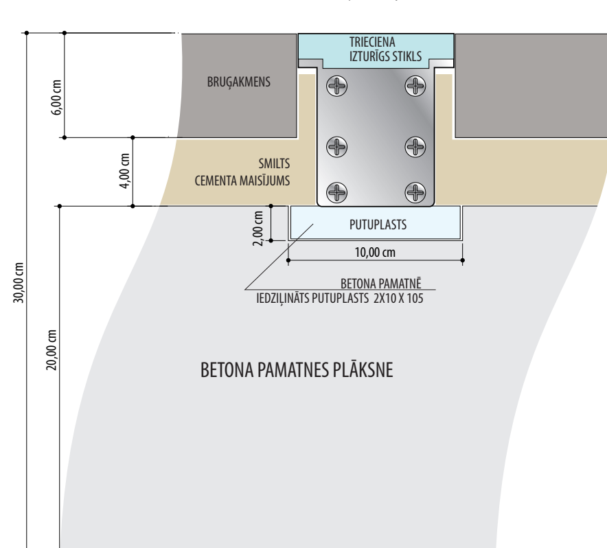
GAISMAS ĶERMEŅA MONTĀŽA. GRIEZUMS
