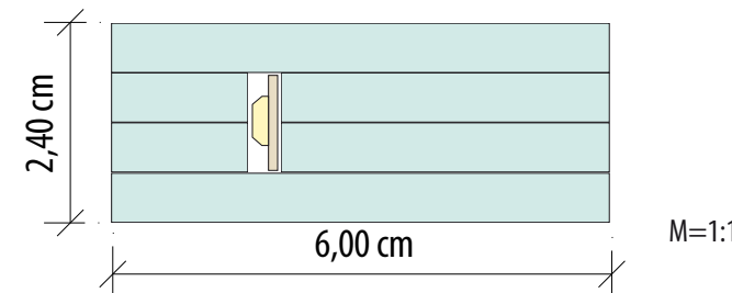
STIKLA PAKETE AR IELĪMĒTU LED DIOŽU SLEJU _2.4X6X150cm
