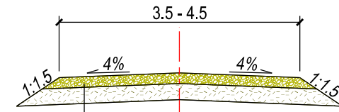
Šķēršprofils nobrauktuvēm Pk 18+20 - Pk 29+29
