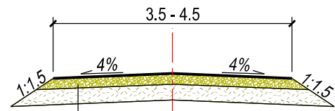
Šķēršprofils nobrauktuvēm Pk 0+00 - Pk 18+20
