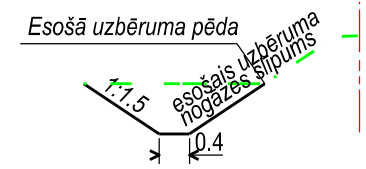
Grāvju rakšana Pk 0+00 - 25+00
