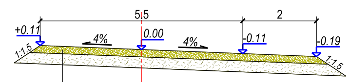
Paplašinājuma vietas šķēršprofils Pk 26+92.63 - Pk
