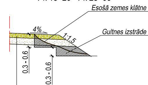
Klātnes paplašināšanas tehnoloģiskā shēma Pk 18+20 - Pk 25+00
